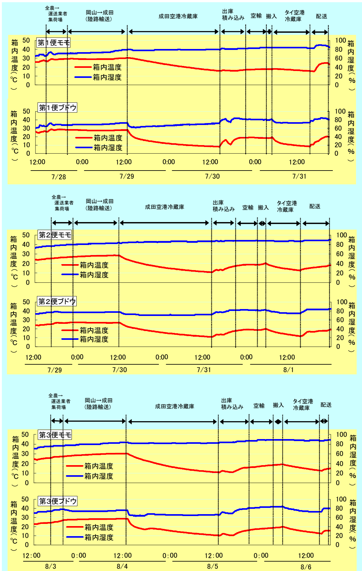
図2 輸送時における箱内の温度、湿度の推移(時刻は日本時間)
