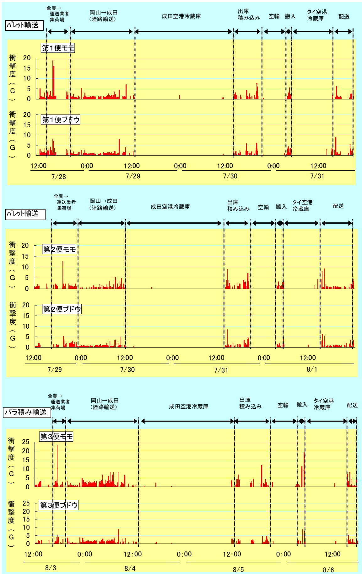
図1 輸送時における果実への衝撃度の推移(時刻は日本時間)
